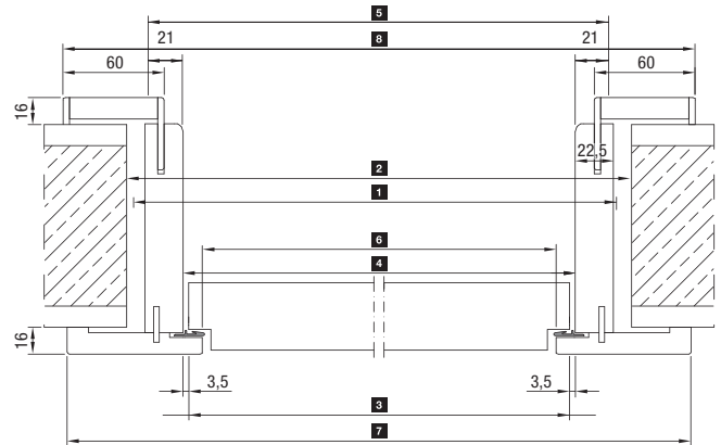
Coupes horizontales
