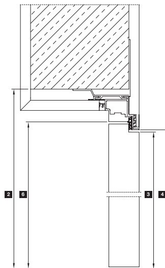
Dimensionnement huisserie Zeroline
