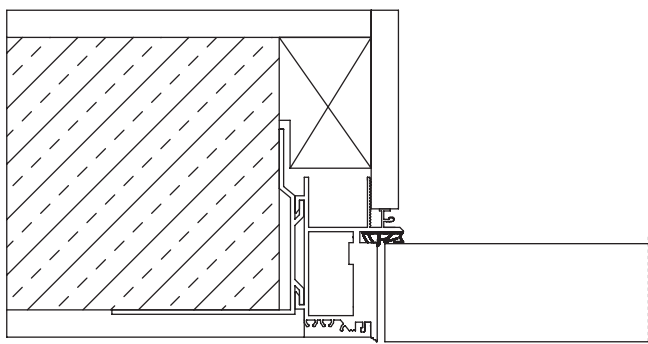
Coupe horizontale avec porte à vantail affleurant
