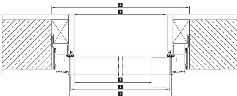
Coupe horizontale avec panneau de porte affleurant
