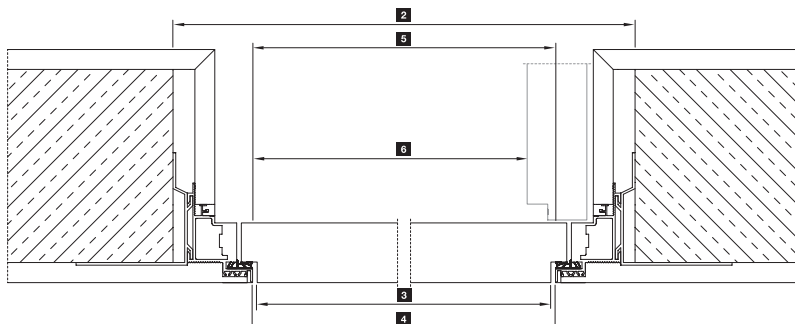
Coupe horizontale avec panneau de porte à ouverture inversée
