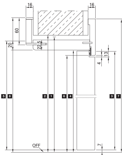
Coupe verticale
