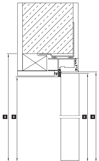
Coupe verticale avec panneau de porte affleurant
