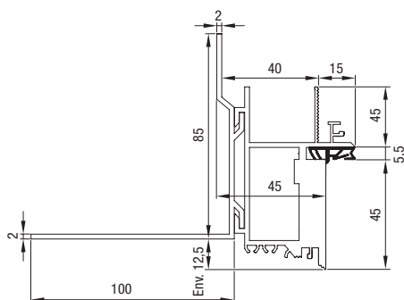
Dimensionnement huisserie Zeroline
